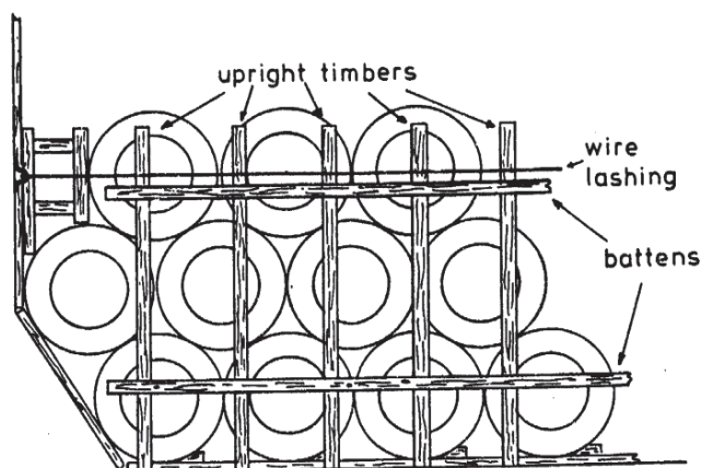
Σχήμα 5 : Ασφάλιση της τελευταίας σειράς στο ανώτατο μέρος έναντι προωραίας και πρυμναίας μετατόπισης
