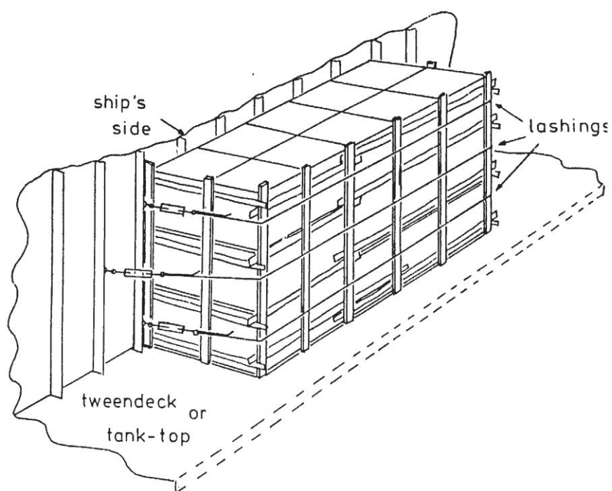
Σχήμα 2 : Ασφάλιση των μονάδων που αποθηκεύονται / στοιβάζονται στην πλευρά του πλοίου.
