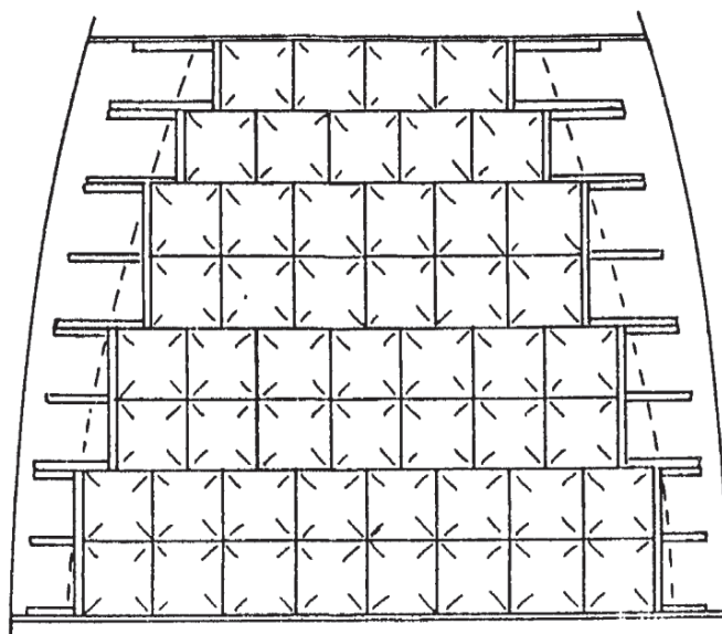
Σχήμα 1: Αποθήκευση/ στοιβάσια των μονάδων φορτίων σε περιοχή στοιβάσιας κωνικού σχήματος ( όπως φαίνεται από ψηλά)
