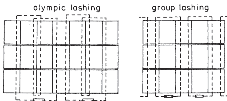
Σχήμα 4 »Στερέωση ανώτερου επιπέδου έναντι προωραίας και πρυμναίας μετατόπισης (θέα από το άνω μέρος )
