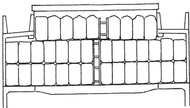
Σχήμα 1: Στοιβάσια FIBCs με υποστυλωμένα διάκενα στο κέντρο της περιοχής αποθήκευσης
