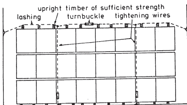
Σχήμα 6: Ασφάλιση της τελευταίας σειράς στο ανώτατο μέρος έναντι προωαίας και πρυμναίας μετατόπισης
